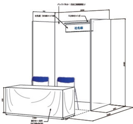
■基礎小間(W1800xH2400xD1800)
